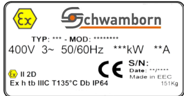
Beispiel Typenschild
